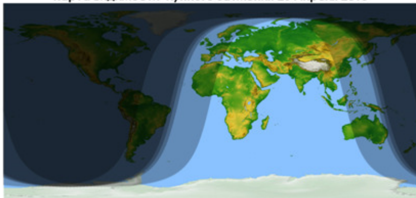
Карта видимости лунного затмения 25 Апреля 2013
