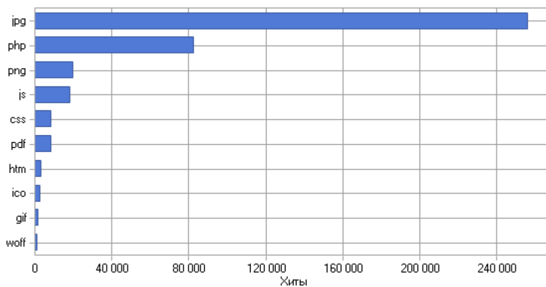
Наиболее запрашиваемые типы файлов
